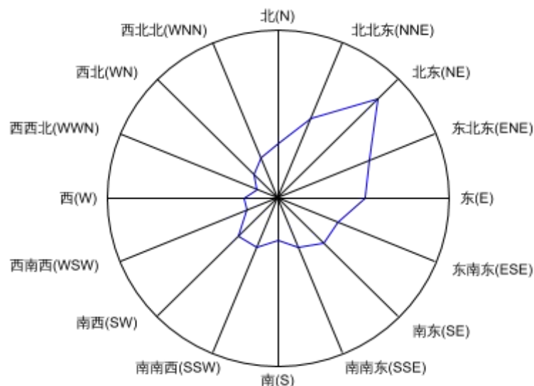
图 5-1 风向玫瑰图
