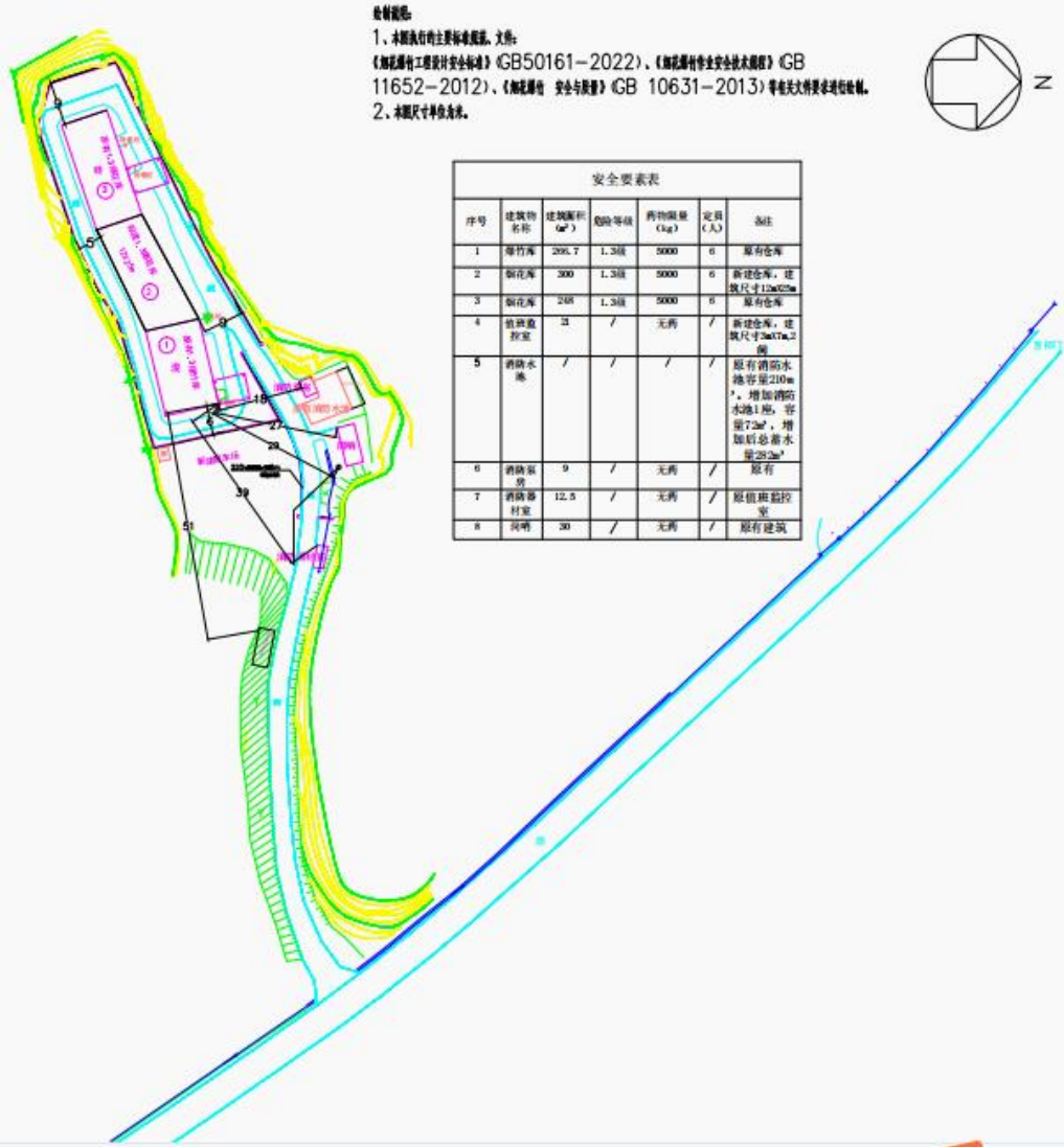
祁门县阊虹烟花爆竹有限责任公司烟花爆竹仓库改扩建项目总平面布置安全距离示意图
